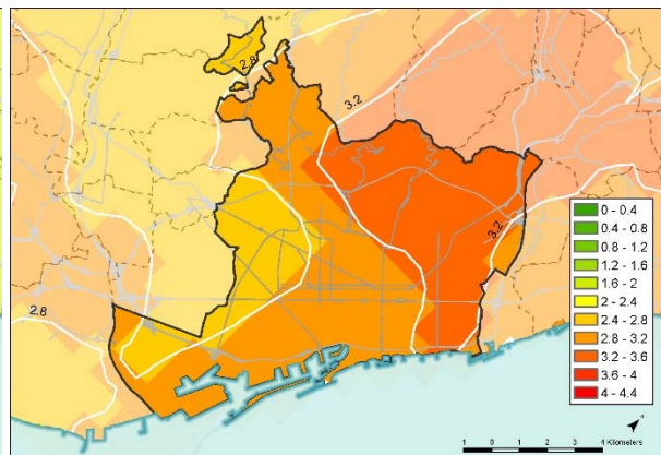
Variació projectada de la temperatura mínima anual respecte al període de referència 1971 – 2000 a Barcelona per al període 2071 – 2100 en l'escenari RCP 8.5
