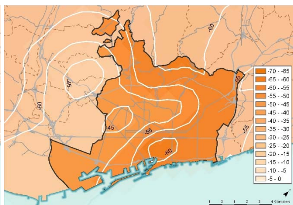
Variació projectada de la Precipitació Mitjana d'estiu respecte al període de referència 1971 – 2000 a Barcelona per al període 2071 – 2100 en l'escenari RCP 8.5
